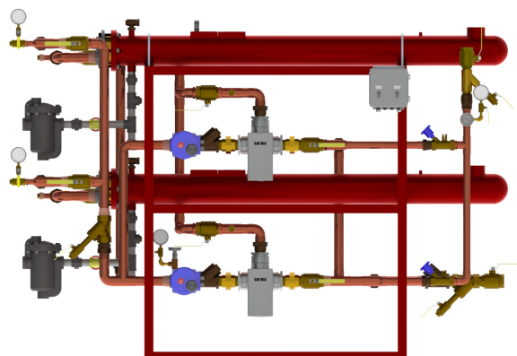
DF665DWP50-50 Double Wall
